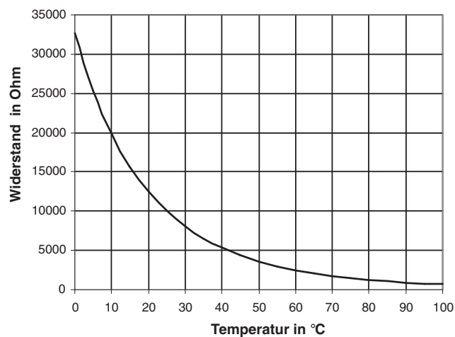
Widerstandskurve Fühler NTC 10 kOhm
