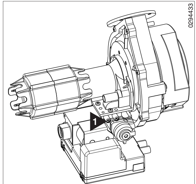
Gasanschlussdruck prüfen
