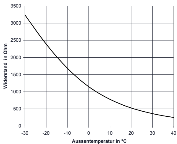
Widerstandskurve Außenfühler
