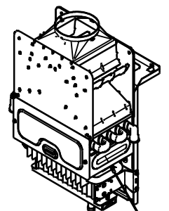
Brennkammer
